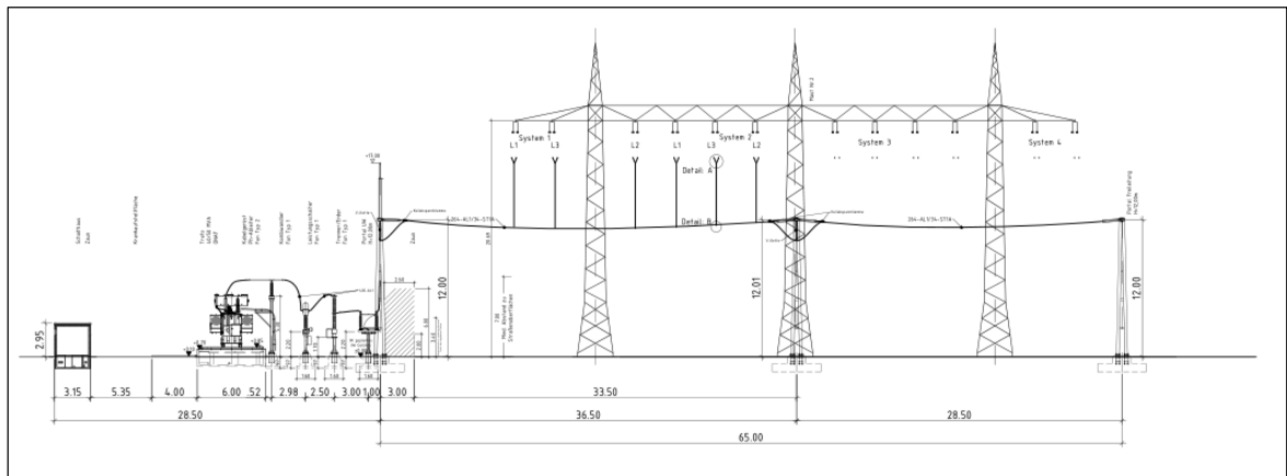
Abbildung 2: Querschnitt geplantes Umspannwerk /6/
