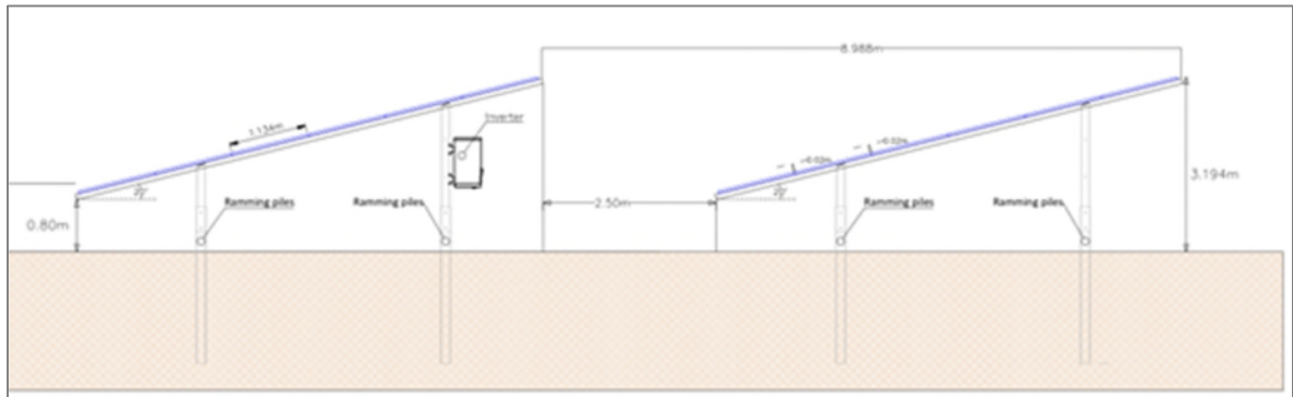
Abbildung 1: Schematische Aufstellung /7/
